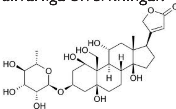
Strukturformel för ouabain
